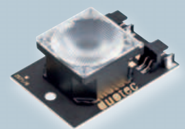
SMD auf Metallkern-Leiterplatte
